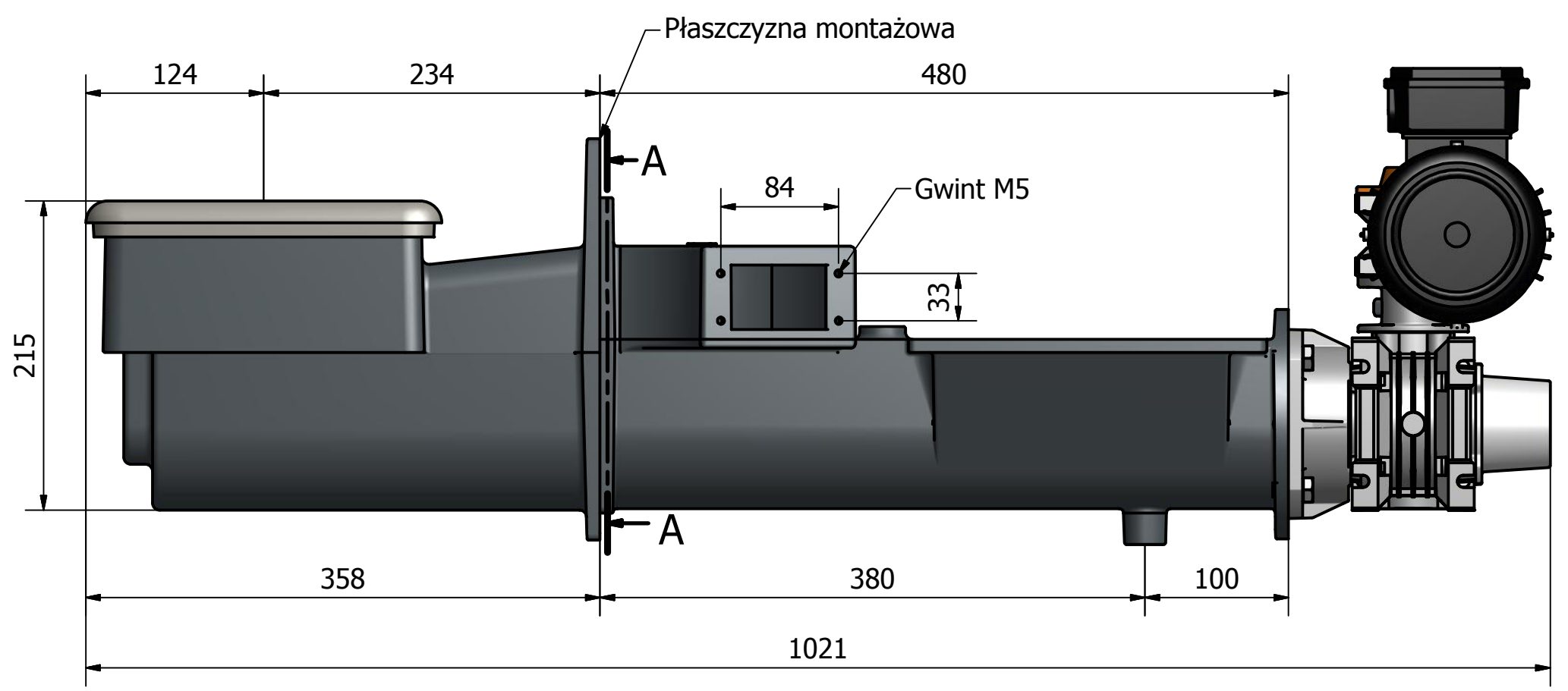
Palnik 25kW
